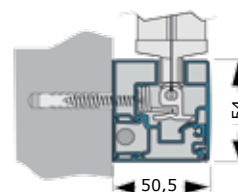
Dimensioner på sideskinne
